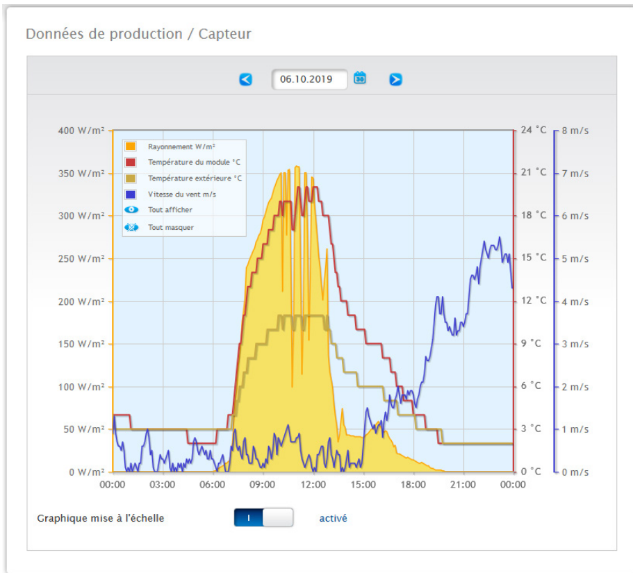
Fig. : Graphique Valeurs de la Sensorbox
