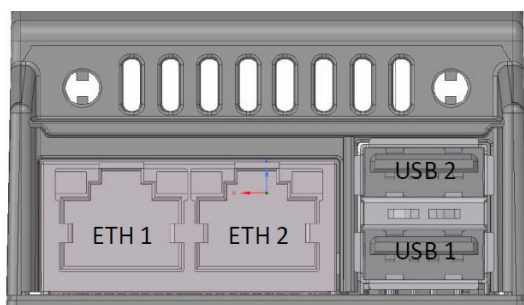
Fig. : Connexions Solar-Log 15 Base – partie inférieure
