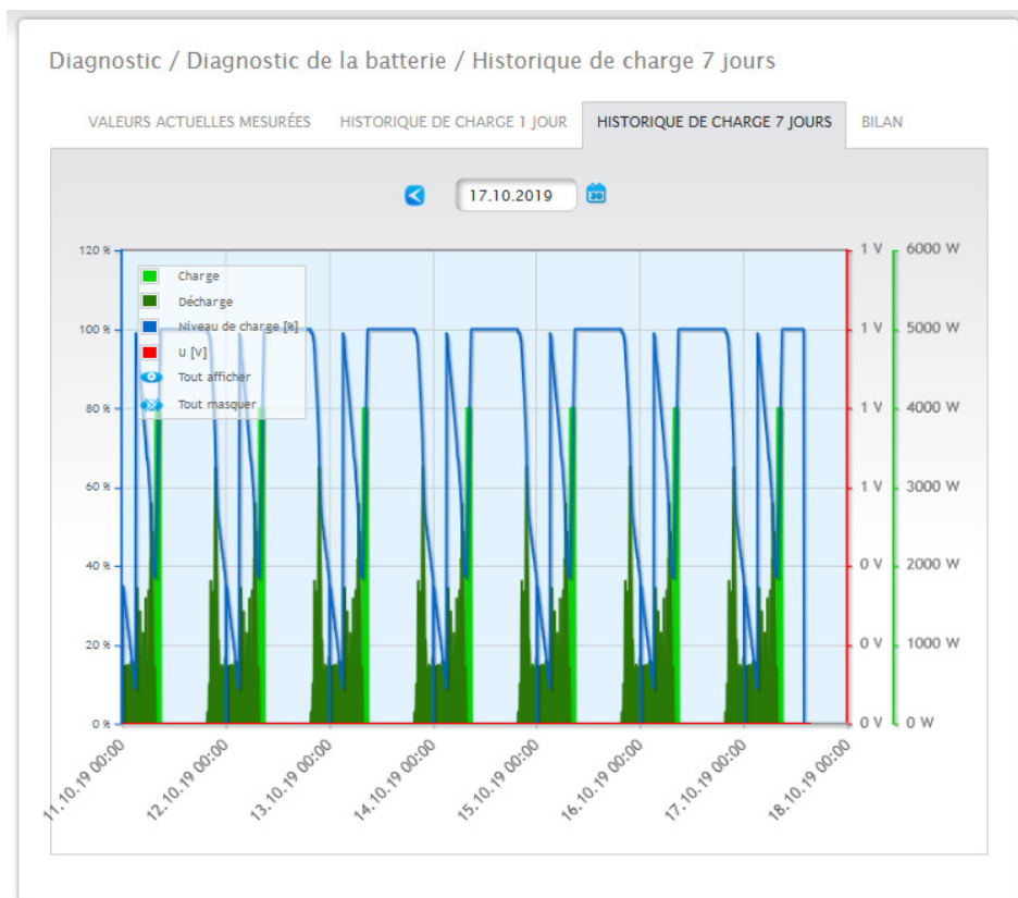
Fig. : Diagnostic de la batterie - Historique de charge 7 jours
