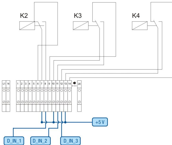
Fig. : Câblage récepteur centralisé avec 3 relais - 3ème exemple
