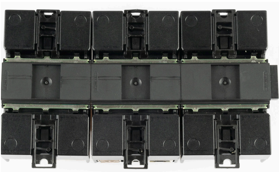
Fig. : Combinaison Solar-Log Base avec Solar-Log MOD I/O et Solar-Log MOD 485 (Connecté - face arrière)
